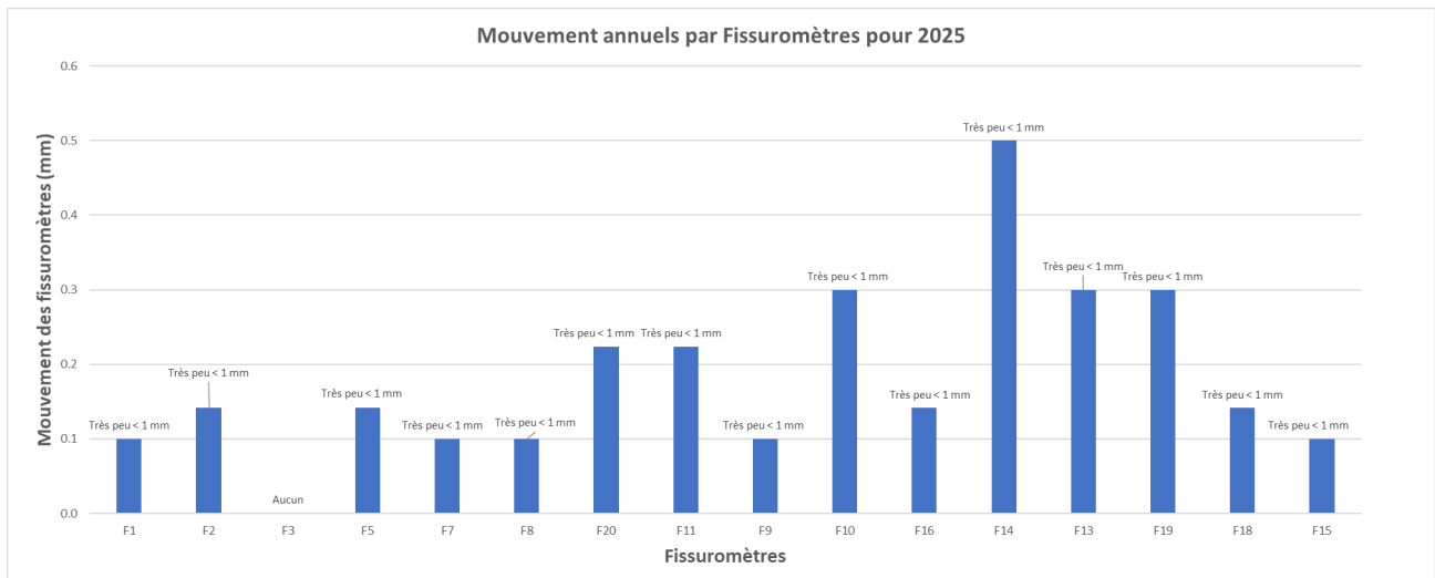
Figure 5 - Histogramme du type de mouvements annuels par fissuromètre pour 2025
