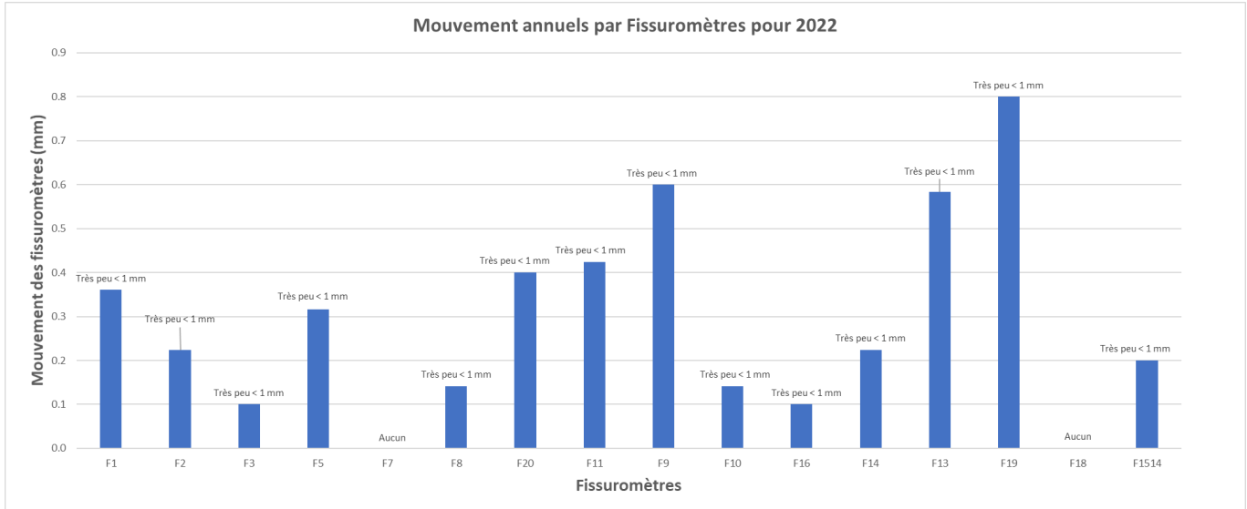
Figure 5 - Histogramme du type de mouvements annuels par fissuromètre pour 2022
