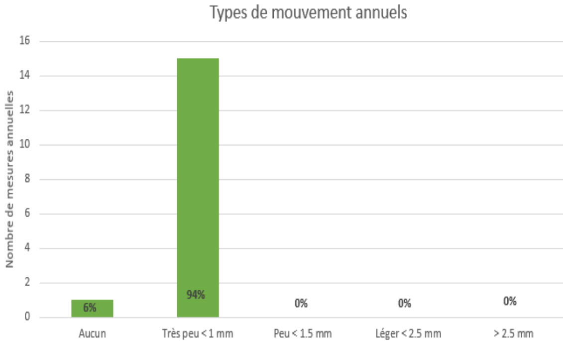
Figure 6 - Histogramme des types de mouvements annuels des fissuromètres
