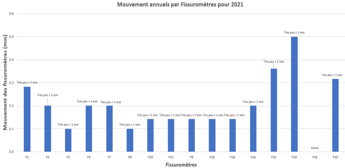
Figure 5 - Histogramme des types de mouvements annuels par fissuromètre pour 2021
