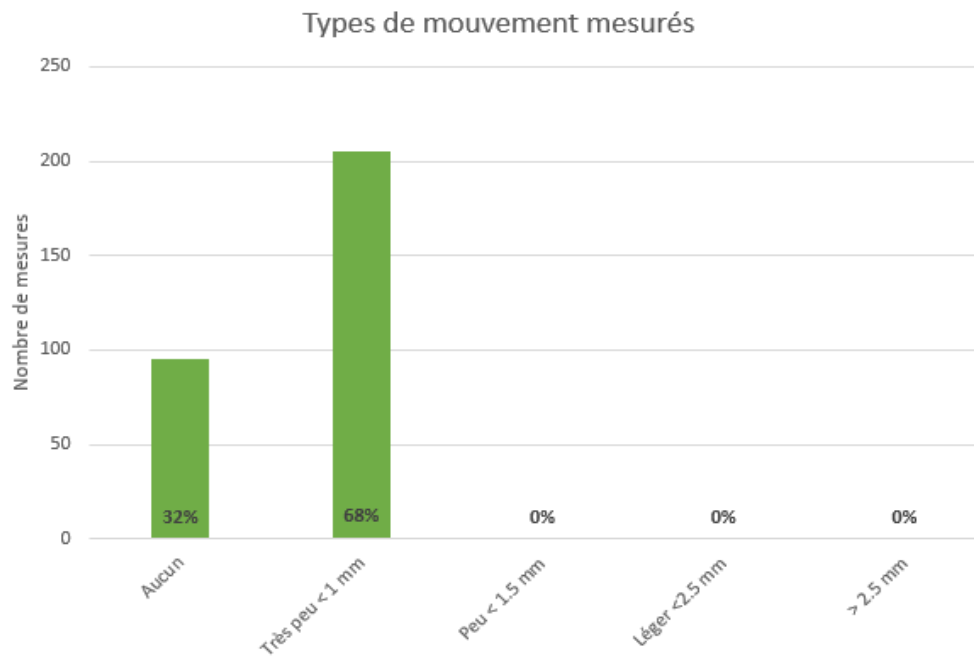
Figure 3 - Histogramme des types de mouvement mesurés aux deux semaines
